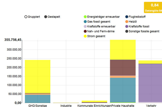
Abbildung 2: Treibhausgasemissionen in t CO 2 -Äquivalente nach Sektoren und Energieträgern für 2017
